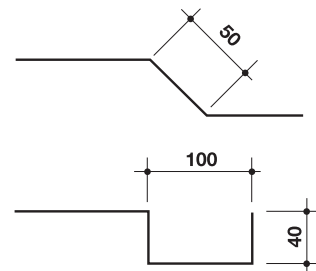
Formas mínimas de plegado (mm).
