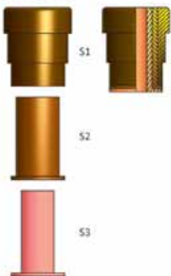
Detalle junta
